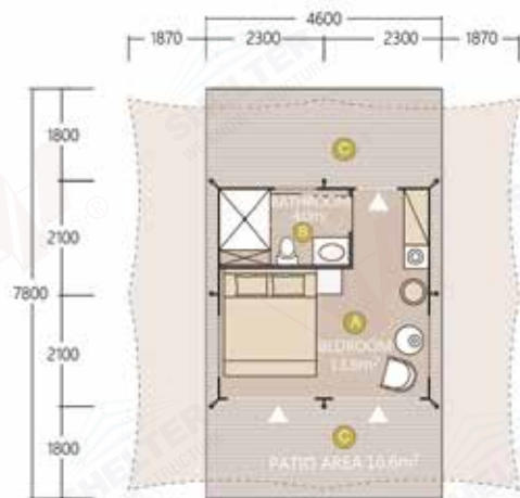
戶型 A Design A
