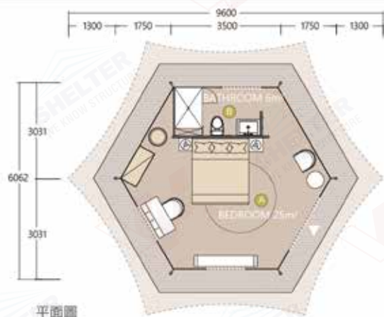
平面圖 Floor Plan
